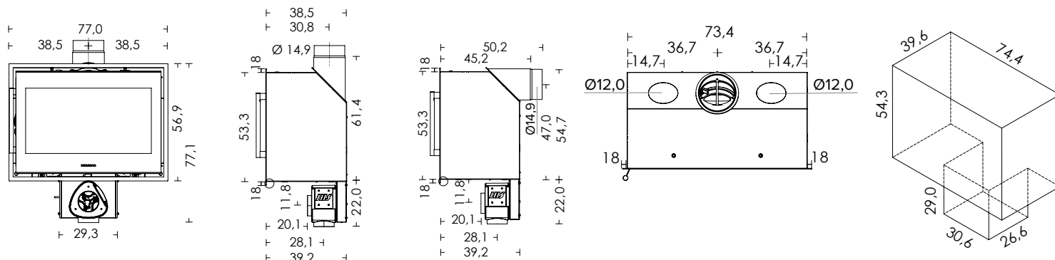
HWAM I 40/55c Türanschlag links, Standardrahmen
