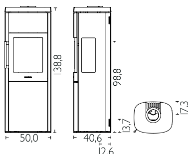
HWAM 4550m mit Seitenscheiben
