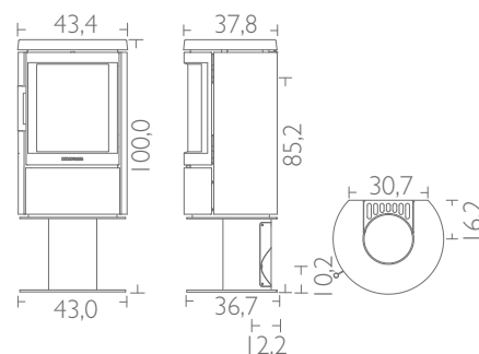
HWAM 2620c auf Säulenfuß
