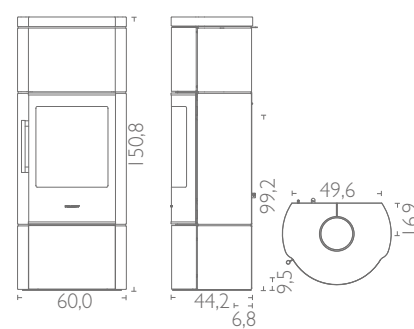
HWAM 3660m mit Specksteinverkleidung
