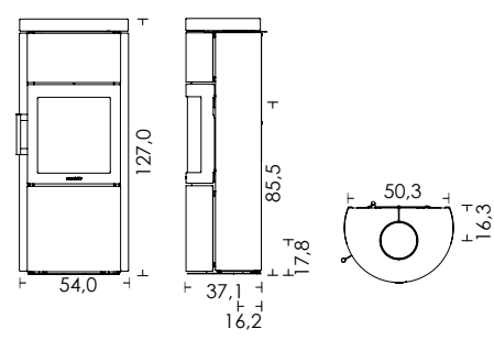
HWAM 3520c mit Specksteinverkleidung
