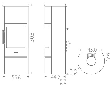
HWAM 3660m, weiß
