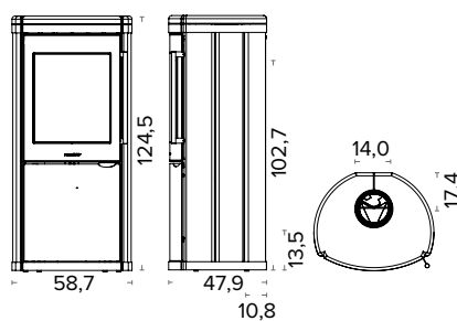
HWAM 4340 mit Rosewood Natursteinverkleidung
