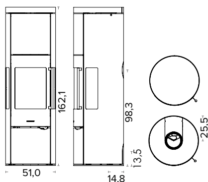
HWAM 4150 mit Seitenscheiben
